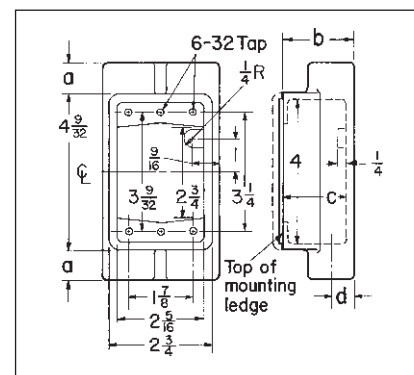
FSCT, FSX, FST, FSCD
